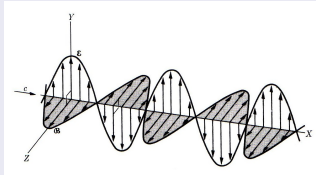
Champs électrique \vec{E} et magnétique \vec{B} dans le cas d'une onde électromagnétique plane polarisée rectilignement
